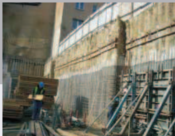
Zabezpieczenie głębokiego wykopu Filharmonia, Kielce
